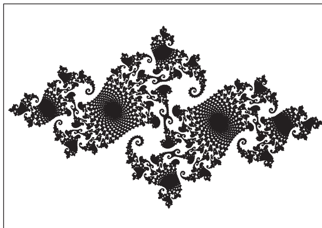
0.3. ábra. Julia-halmaz.
